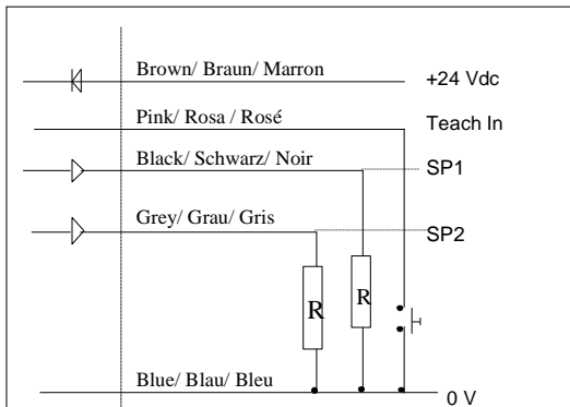
Wiring/Anschlüsse/Raccordement électrique
