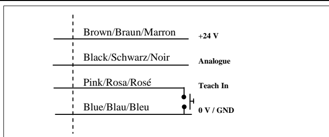
Wiring/Anschlüsse/Raccordement électrique
