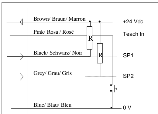
Wiring/Anschlüsse/Raccordement électrique
