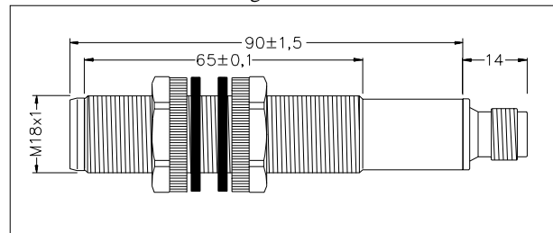
Dimensions / Abmessungen / Dimensions mm
